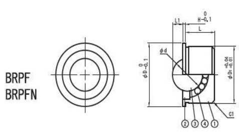
不锈钢本体
